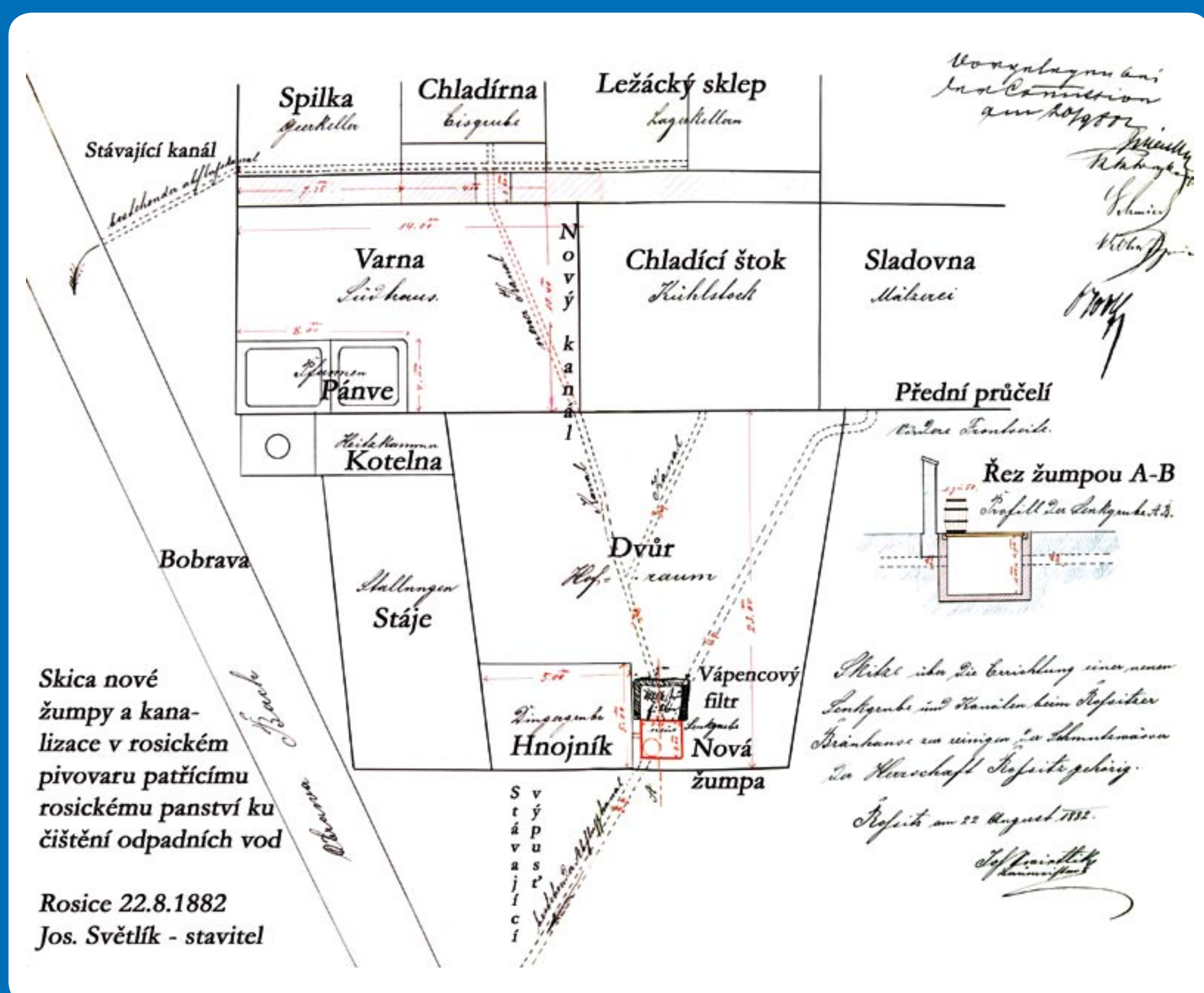
Půdorys stavby pivovaru * Ground plan of the brewery building * Grundriss des Brauereigebäudes
