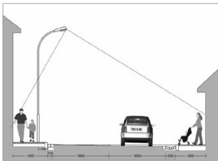
Vzorový řez
