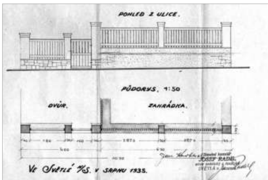
Plánek oplocení
